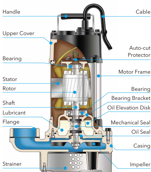
Open Impeller
